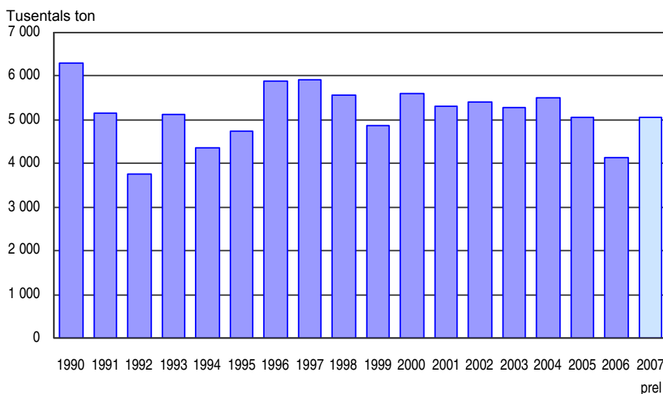
Diagram 2. Spannmål. Totalskördar 1990-2007
